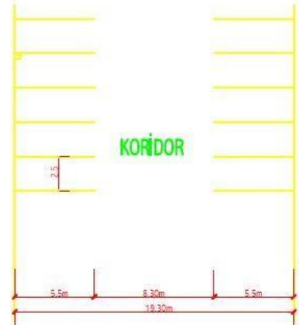
90 derecelik simetrik park hali
