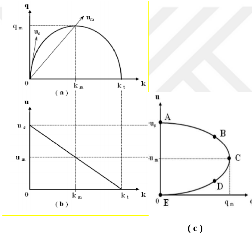
Şekil 3.1.(a). Akım-Yoğunluk, (b). Hız-Yoğunluk, (c). Hız-Akım (Yayla 2011)
