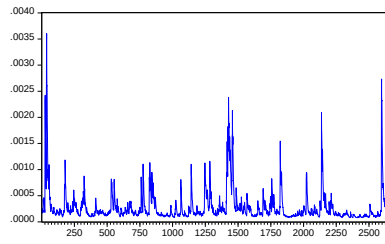
DEĞİŞEN VARYANS P17 (DCC)
