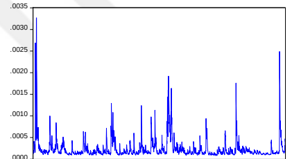
DEĞİŞEN KOVARYANS P18PM (DCC)
