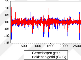
P23 GERÇEKLEŞEN GETİRİ ve BEKLENEN GETİRİ (CCC)
