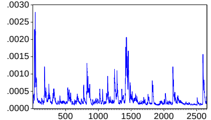
DEĞİŞEN KOVARYANS P12PM (DCC)
