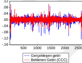
P22 GERÇEKLEŞEN GETİRİ ve BEKLENEN GETİRİ (CCC)
