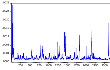
DEĞİŞEN VARYANS P25 (CCC)
