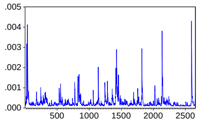
DEĞİŞEN VARYANS P13 (DCC)
