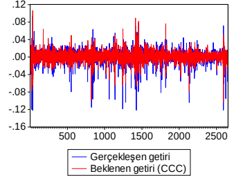
P30 GERÇEKLEŞEN GETİRİ ve BEKLENEN GETİRİ (CCC)
