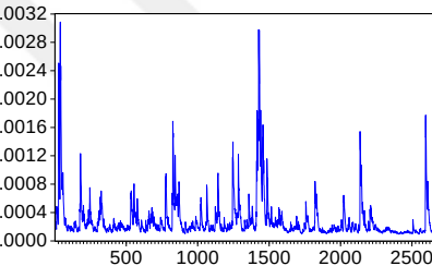
DEĞİŞEN VARYANS P12 (DCC)
