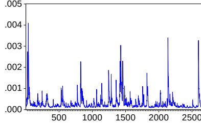
DEĞİŞEN VARYANS P4 (DCC)
