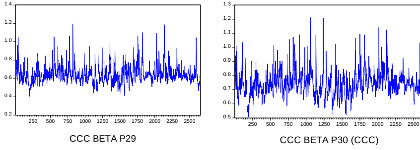
Şekil 4.27 CCC Yöntemine Göre Portföylerin Koşullu Betaları
