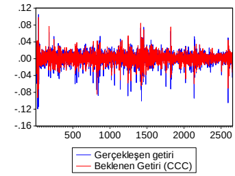
P18 GERÇEKLEŞEN GETİRİ ve BEKLENEN GETİRİ (CCC)
