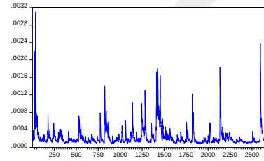
DEĞİŞEN KOVARYANS P16PM (DCC)
