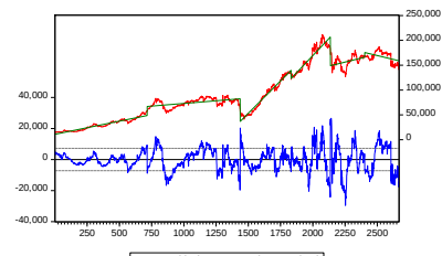
P18 KIRILMA NOKTALARI
