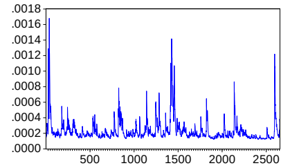
DEĞİŞEN KOVARYANS P6PM (CCC)
