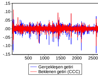
P16 GERÇEKLEŞEN GETİRİ ve BEKLENEN GETİRİ (CCC)
