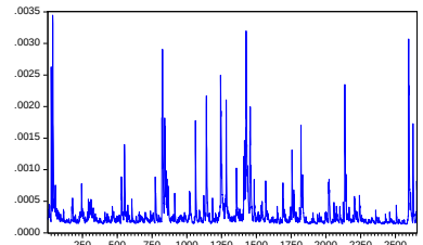
DEĞİŞEN VARYANS P27 (CCC)
