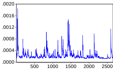
DEĞİŞEN KOVARYANS P7PM (CCC)
