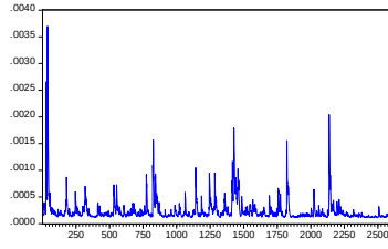
DEĞİŞEN VARYANS P29 (CCC)
