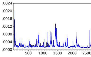
DEĞİŞEN KOVARYANS P8PM (CCC)
