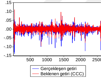
P26 GERÇEKLEŞEN GETİRİ ve BEKLENEN GETİRİ (CCC)
