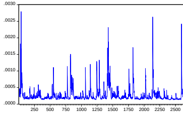
DEĞİŞEN VARYANS P28 (CCC)
