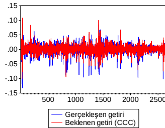
P29 GERÇEKLEŞEN GETİRİ ve BEKLENEN GETİRİ (CCC)
