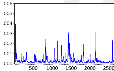
DEĞİŞEN VARYANS P10 (DCC)
