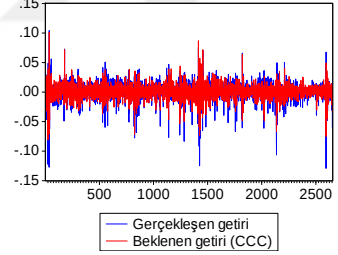
P27 GERÇEKLEŞEN GETİRİ ve BEKLENEN GETİRİ (CCC)
