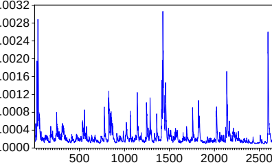
DEĞİŞEN VARYANS P6 (DCC)
