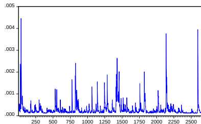
DEĞİŞEN VARYANS P16 (DCC)
