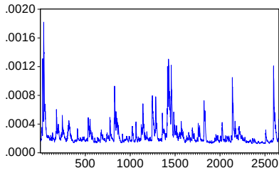
DEĞİŞEN KOVARYANS P4PM (CCC)
