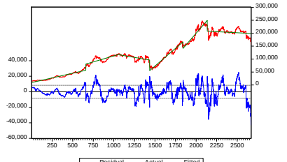
P17 KIRILMA NOKTALARI
