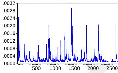
DEĞİŞEN VARYANS P7 (DCC)
