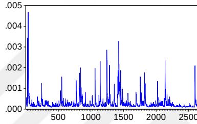
DEĞİŞEN VARYANS P8 (DCC)
