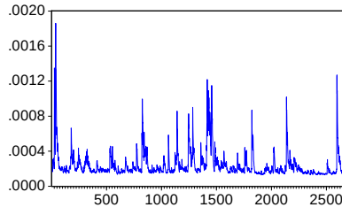
DEĞİŞEN KOVARYANS P5PM (CCC)
