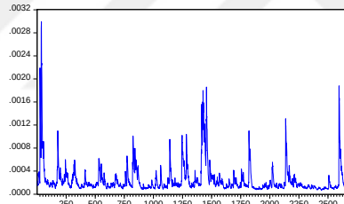
DEĞİŞEN KOVARYANS P17PM (DCC)
