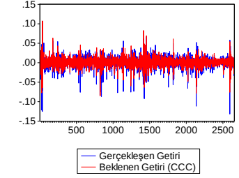
P21 GERÇEKLEŞEN GETİRİ ve BEKLENEN GETİRİ (CCC)
