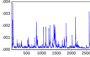
DEĞİŞEN VARYANS P5 (DCC)
