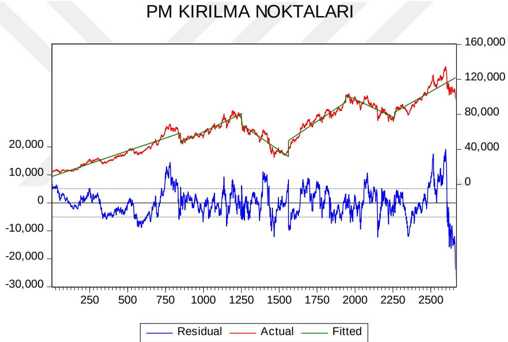
Şekil 4.3 02.01.2003 - 29.08.2013 Tarihleri Arasında Gerçekleşen PM Kırılmaları
