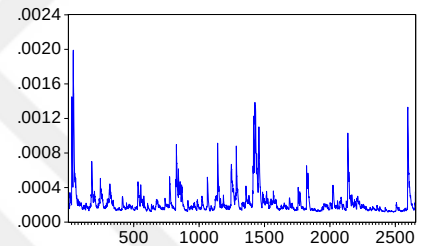
DEĞİŞEN KOVARYANS P3PM (CCC)
