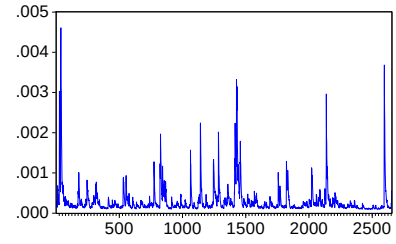
DEĞİŞEN VARYANS P3 (DCC)
