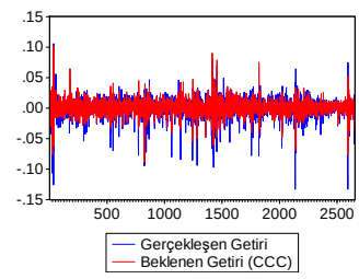
P19 GERÇEKLEŞEN GETİRİ ve BEKLENEN GETİRİ (CCC)
