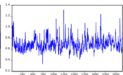
DCC BETA P21
