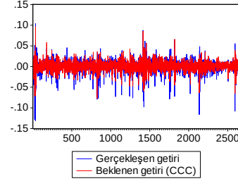
P17 BEKLENEN GETİRİ ve GERÇEKLEŞEN GETİRİ (CCC)
