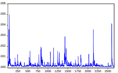
DEĞİŞEN VARYANS P18 (DCC)
