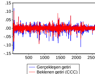
Şekil 4.28 Portföylerin Gerçekleşen Getirileri ve CCC Yöntemine Göre Beklenen Getirileri
