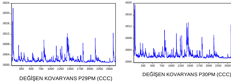
Şekil 4.26 CCC Yöntemine Göre Portföylerin Koşullu Kovaryansları
