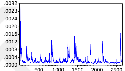
DEĞİŞEN KOVARYANS P15PM (DCC)
