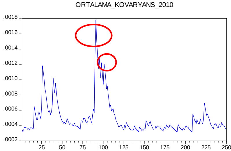
Şekil 4.16 02.01.2010-31.12.2010 Tarihleri Arasında Ortalama Kovaryans
