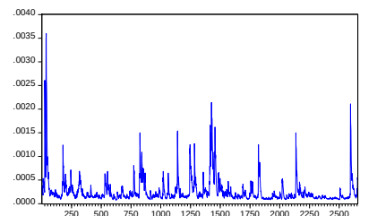
DEĞİŞEN KOVARYANS P24PM (DCC)
