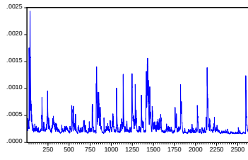
DEĞİŞEN VARYANS P26 (CCC)
