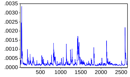
DEĞİŞEN KOVARYANS P9PM (DCC)
