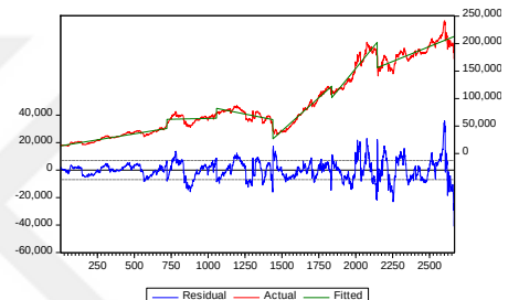
P12 KIRILMA NOKTALARI
