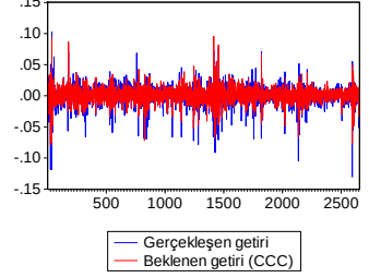
P20 GERÇEKLEŞEN GETİRİ ve BEKLENEN GETİRİ (CCC)
