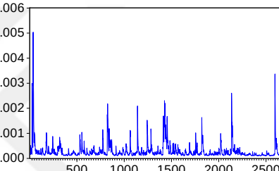
DEĞİŞEN VARYANS P9 (DCC)
