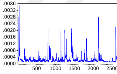
DEĞİŞEN VARYANS P11 (DCC)
