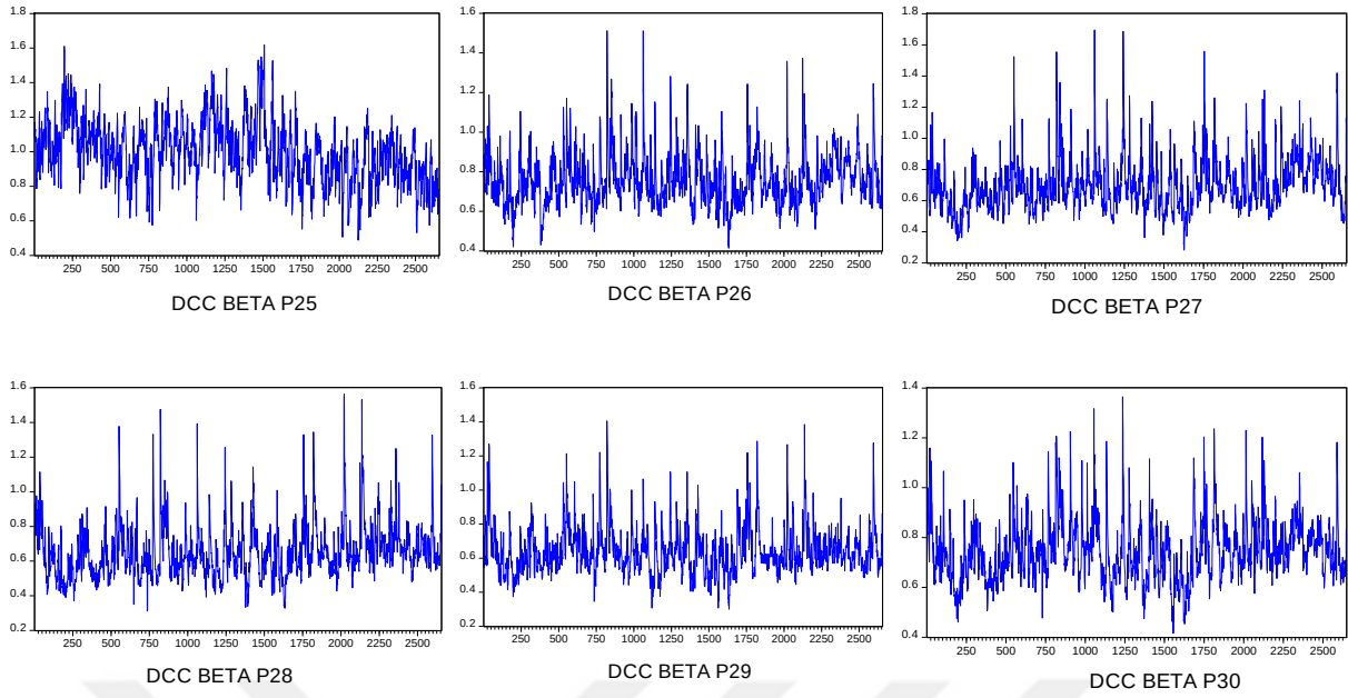
Şekil 4.31 DCC Yöntemine Göre Portföylerin Koşullu Betaları
