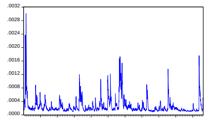
DEĞİŞEN KOVARYANS P21PM (DCC)
