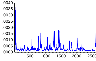
DEĞİŞEN VARYANS P1 (DCC)
