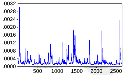
DEĞİŞEN KOVARYANS P13PM (DCC)
