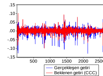
P28 GERÇEKLEŞEN GETİRİ ve BEKLENEN GETİRİ (CCC)
