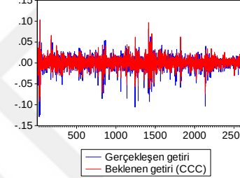
P25 GERÇEKLEŞEN GETİRİ ve BEKLENEN GETİRİ (CCC)
