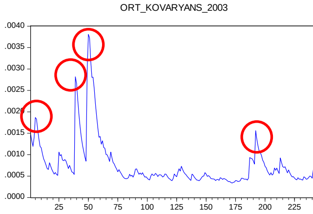
Şekil 4.6 02.01.2003-31.12.2003 tarihleri arasında ortalama kovaryans
