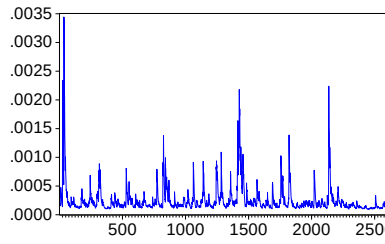
DEĞİŞEN VARYANS P14 (DCC)
