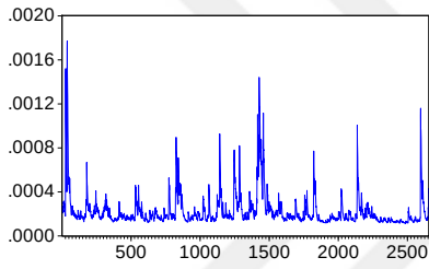
DEĞİŞEN KOVARYANS P1PM (CCC)
