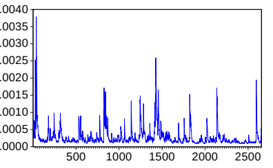
DEĞİŞEN VARYANS P15 (DCC)
