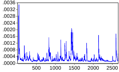
DEĞİŞEN KOVARYANS P10PM (DCC)
