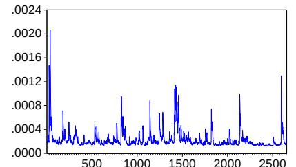
DEĞİŞEN KOVARYANS P9PM (CCC)
