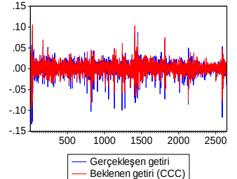
Şekil 4.28 Portföylerin Gerçekleşen Getirileri ve CCC Yöntemine Göre Beklenen Getirileri
