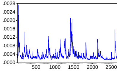
DEĞİŞEN VARYANS PM (DCC)
