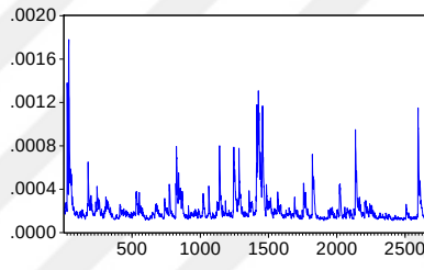
DEĞİŞEN KOVARYANS P2PM (CCC)
