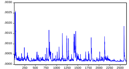
DEĞİŞEN VARYANS P30 (CCC)
