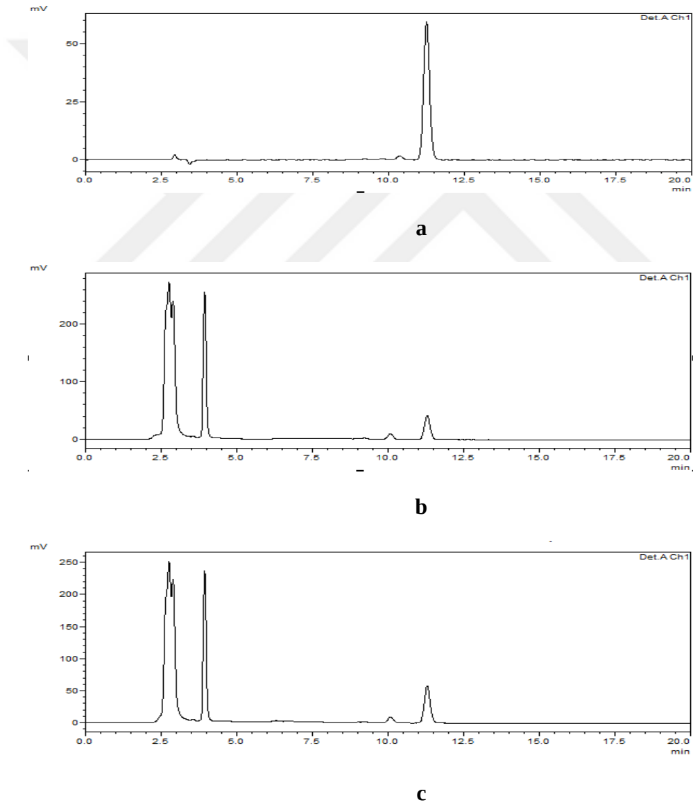
Şekil 3.5. \alpha -tokoferol çalışmalarına ait kromotogramlar (a: 10 ppm konsantrasyondaki standart \alpha -tokoferol, b: örnek, c: örnek+ \alpha -tokoferol)
