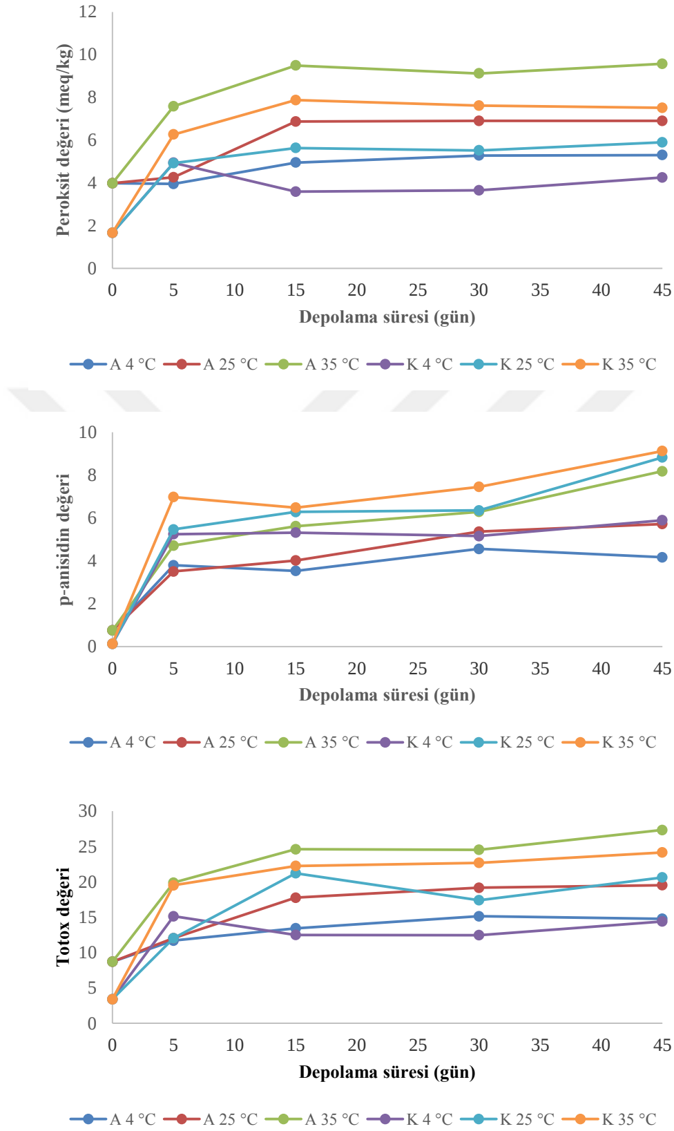
Şekil 4.11. Depolama sıcaklığı ve süresine bağlı olarak mayonezlerin peroksit, p-anisidin ve totox değerlerinin değişimi
