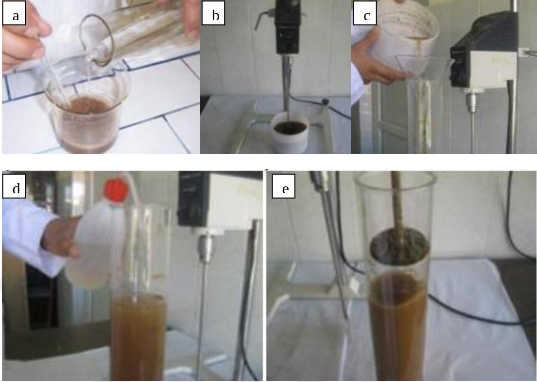
Şekil 3.4. Tekstür analizinin aşamaları a) Harcın hazırlanması; b) Mikserde karıştırma işlemi; c) Sedimantasyon silindirine aktarma işlemi; d) Suyla tamamlama işlemi; e) Karıştırma çubuğuyla süspansiyonun karıştırılması işlemi.
