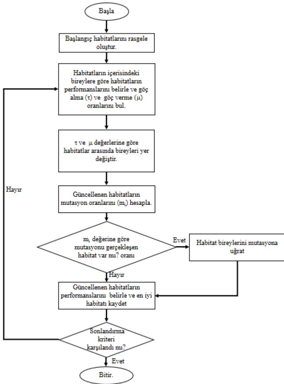
Şekil 3.3. Biyocoğrafya tabanlı optimizasyon yöntemi akış şeması
