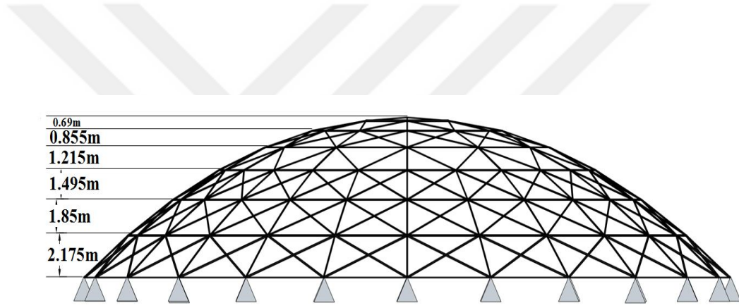
Şekil 4.11. 354 elemanlı uzay kafes kubbe yapının yan görünü
