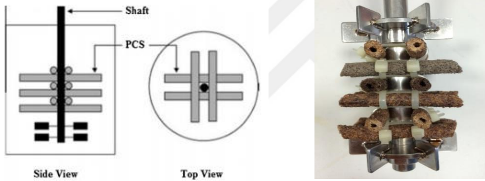
Şekil 3.6. Biyofilm rektör diyagramı.
