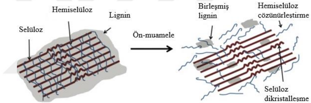
Şekil 2.14. Lignoselülozik polimerlerin matrisinin şematik görünüşü, önişlemin selülozdan hemiselüloz ve lignin'den ayrıldığı (Mosier vd., 2005).
