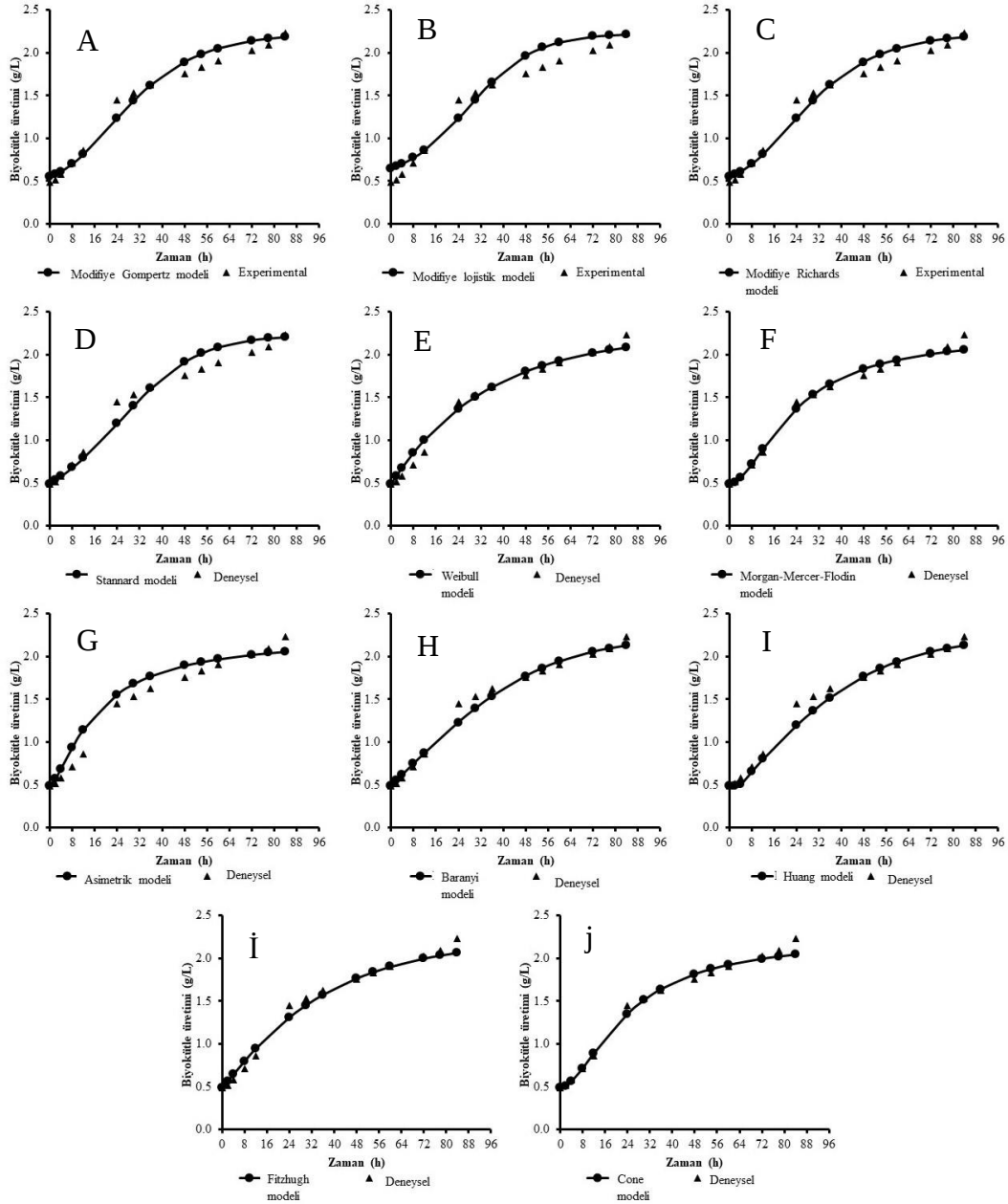
Şekil 4.11. Kullanılan matematiksel modeller ile %75 RH + %25 K + YE + P besiyeri ortamında fit edilen P. stipitis (ATCC 58785) mayasının hücre gelişim eğrileri.
