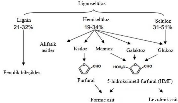
Şekil 2.15. Lignoselülozların hidrolizi ile oluşan inhibitör bileşikler.
