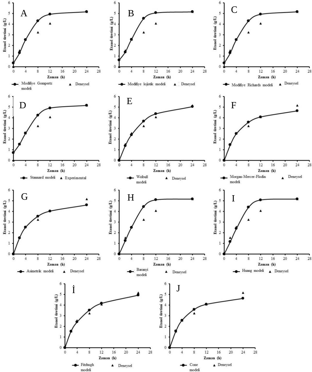
Şekil 4.9. En iyi fermentasyon koşulları altında (%50 RH + %50 G + YE + P besiyeri ortamında) her bir modele ait tahmin edilen etanol değerlerinin deneysel etanol değerleri ile grafike edilmesi.
