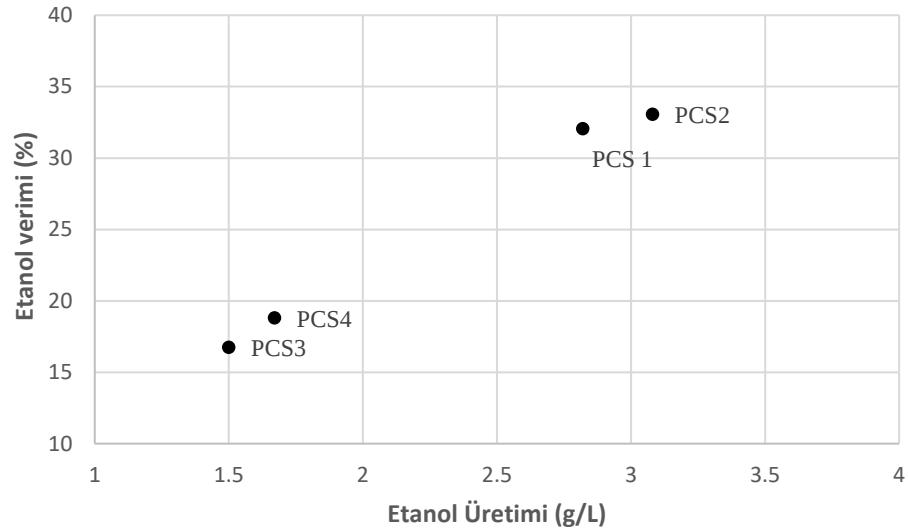
Şekil 4.3. P.stipitis ATCC 58784 ile ksiloz fermentasyonu için etanol üretimi vs etanol üretimi.
