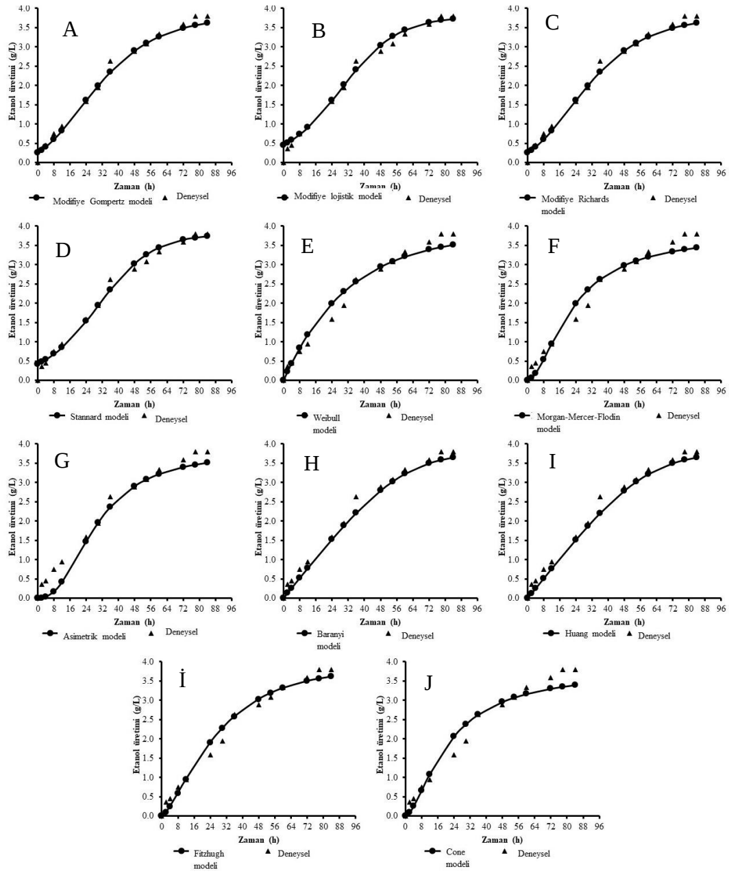
Şekil 4.12. En iyi fermentasyon koşulları altında (%75 RH + %25 K + YE + P besiyeri ortamında) her bir modele ait tahmin edilen etanol değerlerinin deneysel etanol değerleri ile grafike edilmesi.
